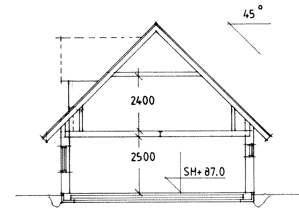
SEKTION
