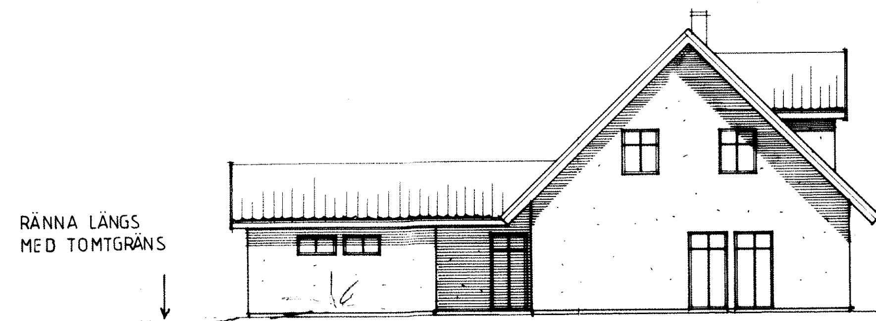
NORDVÄST
