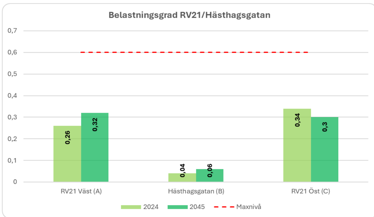
Figur 21. Belastningsgrad korsningspunkt 3.
