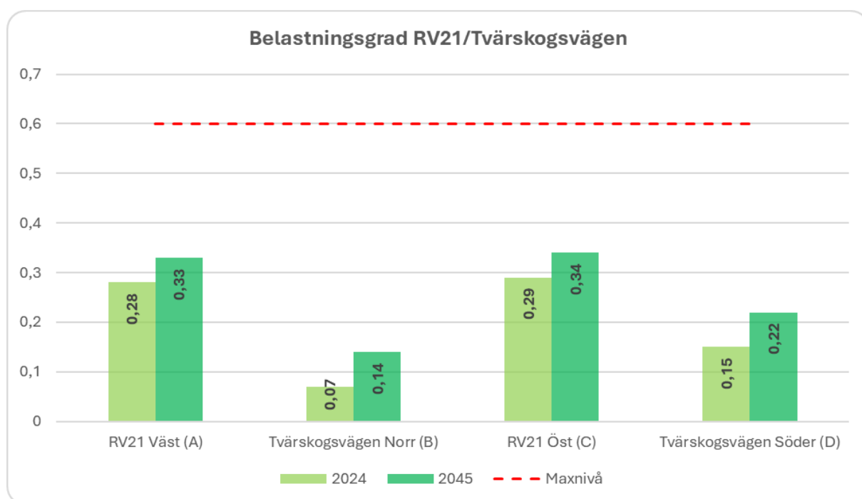
Figur 20. Belastningsgrad, korsningspunkt 2.
