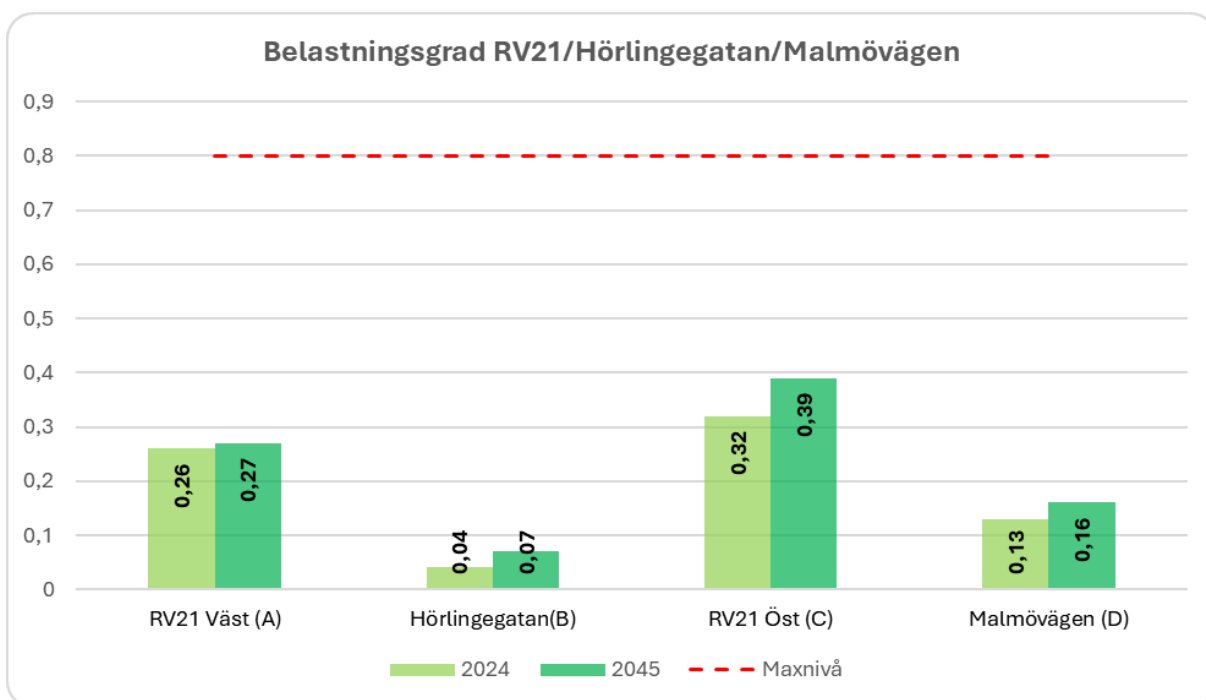
Figur 22. Belastningsgrad korsningspunkt 4.
